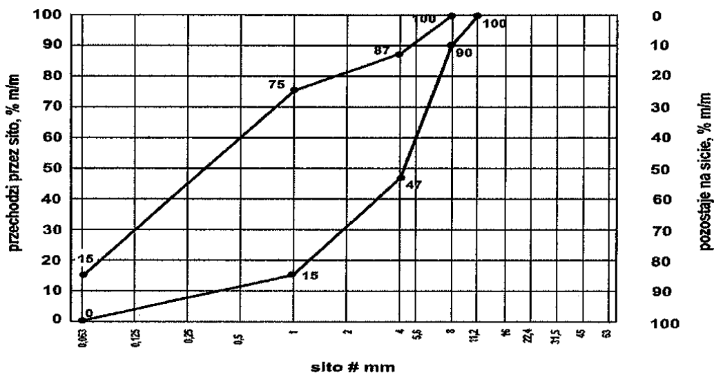
Rys. 1. Krzywe graniczne uziarnienia mieszanki kruszyw 0/8 mm do górnej warstwy podłoża ulepszonych
