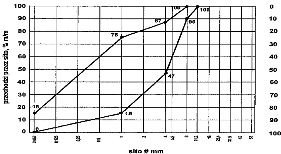
Rys. 1. Krzywe graniczne uziarnienia mieszanki kruszyw 0/8 mm do górnej warstwy podłoża ulepszonego
