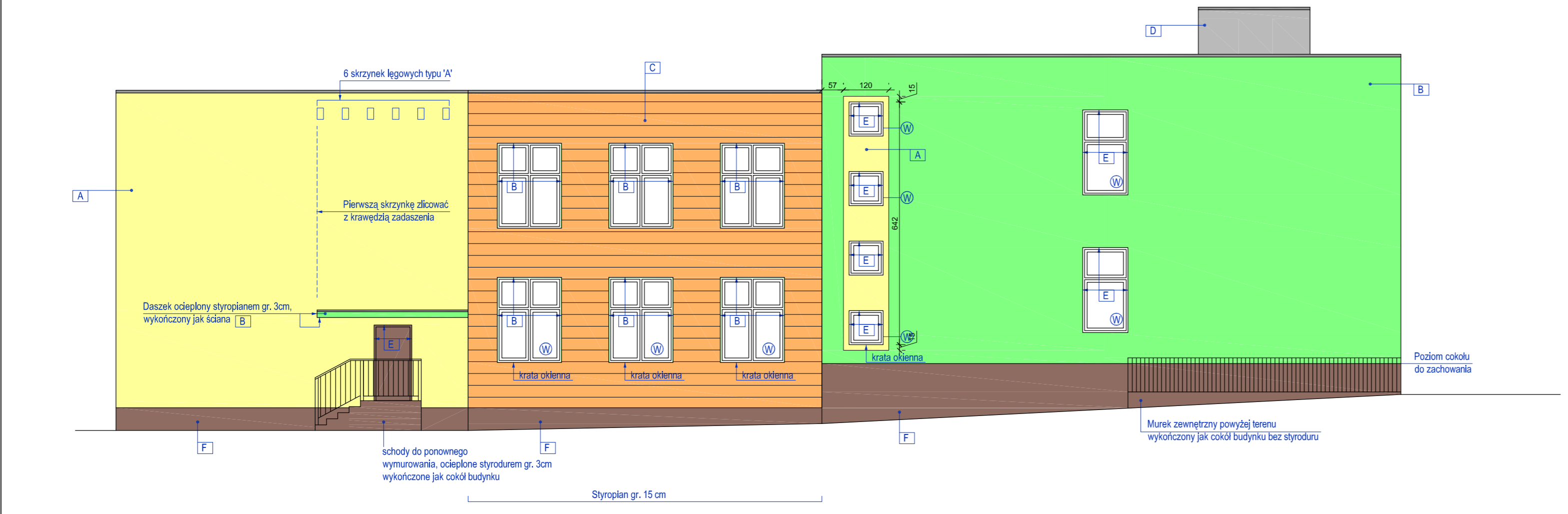
ELEWACJA POŁUDNIOWO-WSCHODNIA (A-C-E-G)
