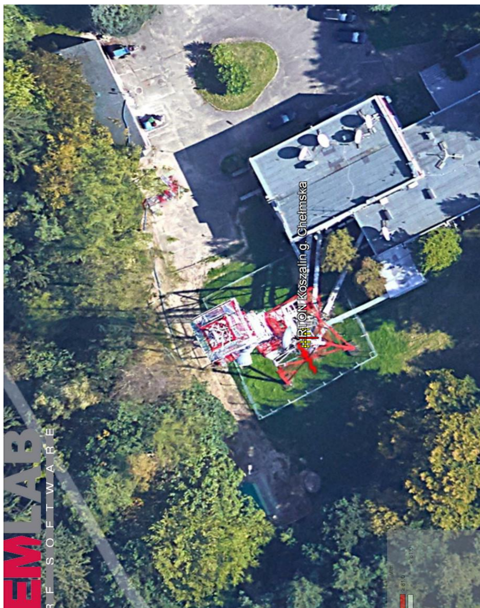
Rys. 2. Rzut poziomy rozkładu pola elektromagnetycznego anteny nowo projektowanej linii radiowej w otoczeniu RTON Koszalin / Góra Chelmska przewidzianej do zainstalowania na wysokości 40 m nad poziomem terenu.
