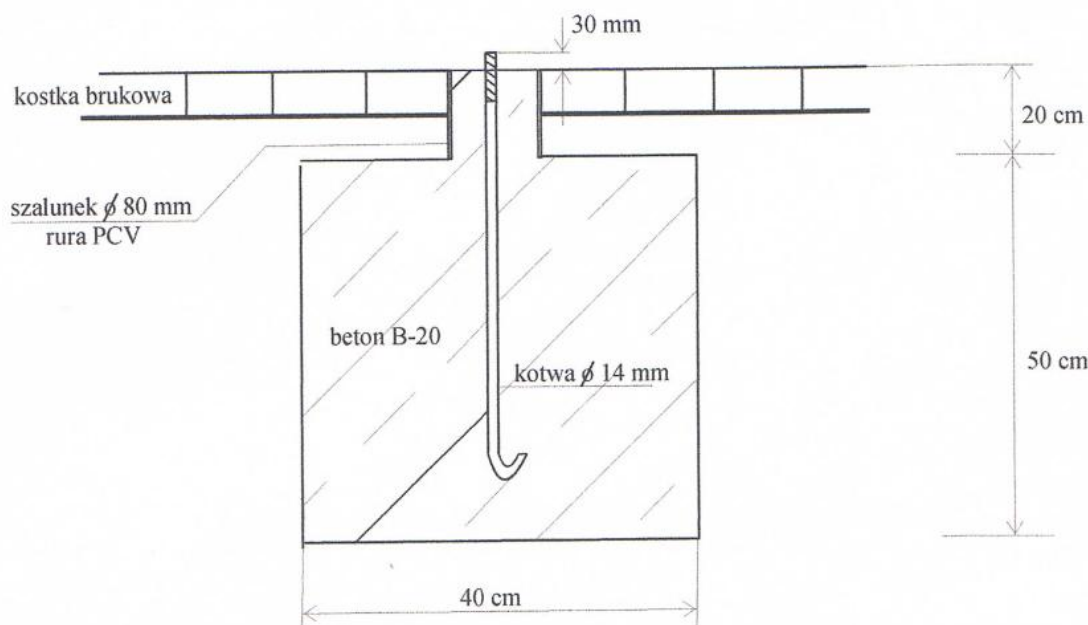
Rys. 2 Szczegół fundamentu punktowego i montażu kotwy stalowej gwintowanej o śr. 14 mm
