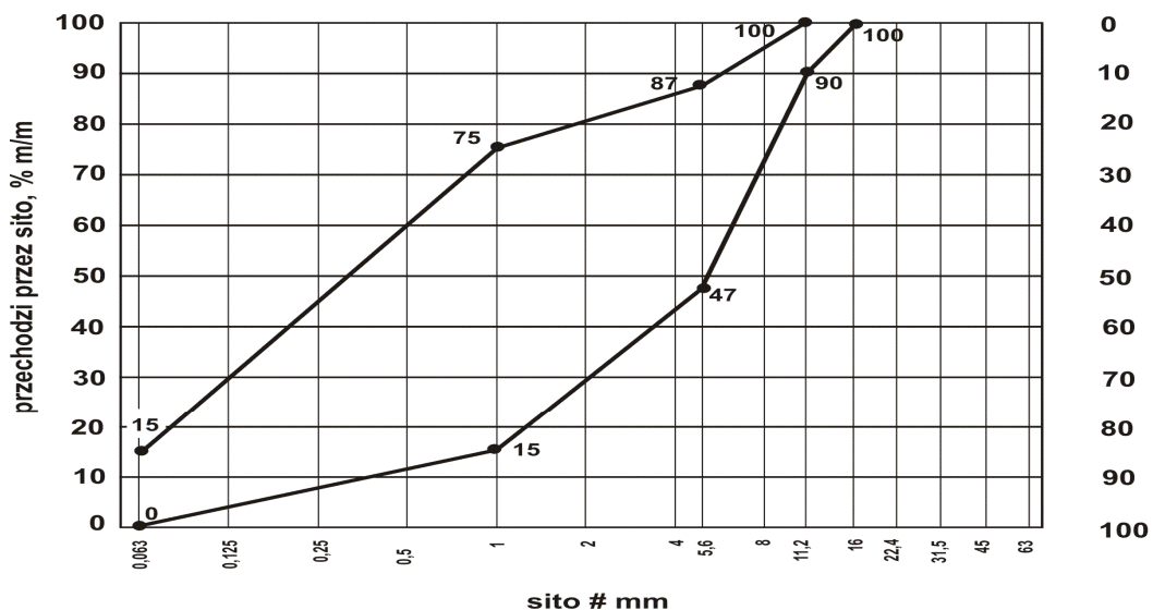
Rys. 2. Uziarnienie mieszanki niezwiązanej 0/11,2 dla warstwy mrozoochronnej
