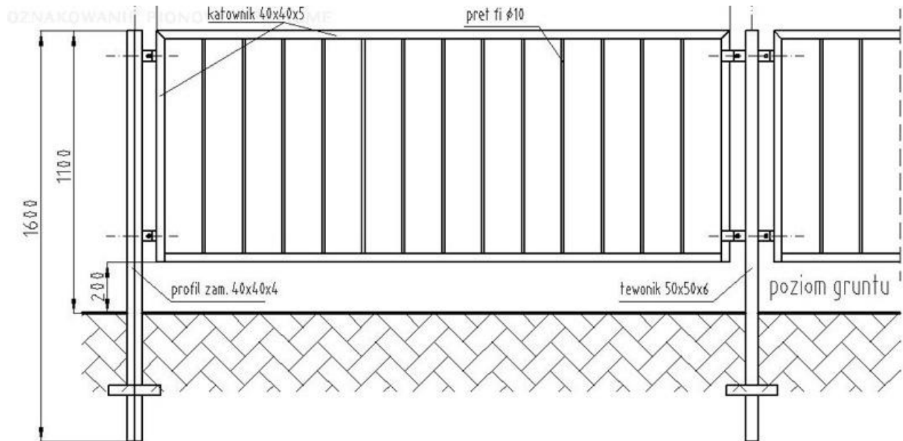
Rys. 1. Balustrady chodnikowe U-11a
