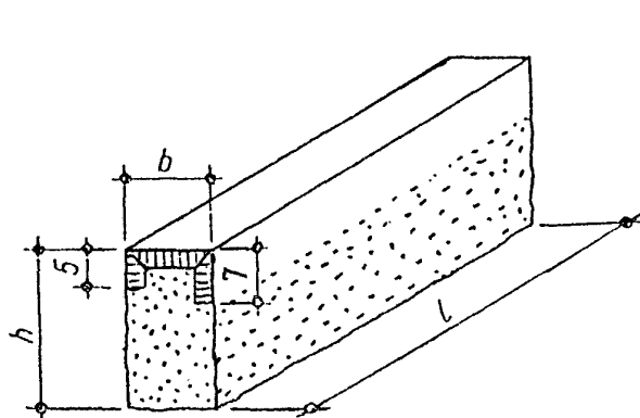
Rys. 5. Krawężnik drogowy rodzaju A
