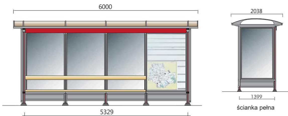
Rys. 1 Widok wiaty przystankowej.
