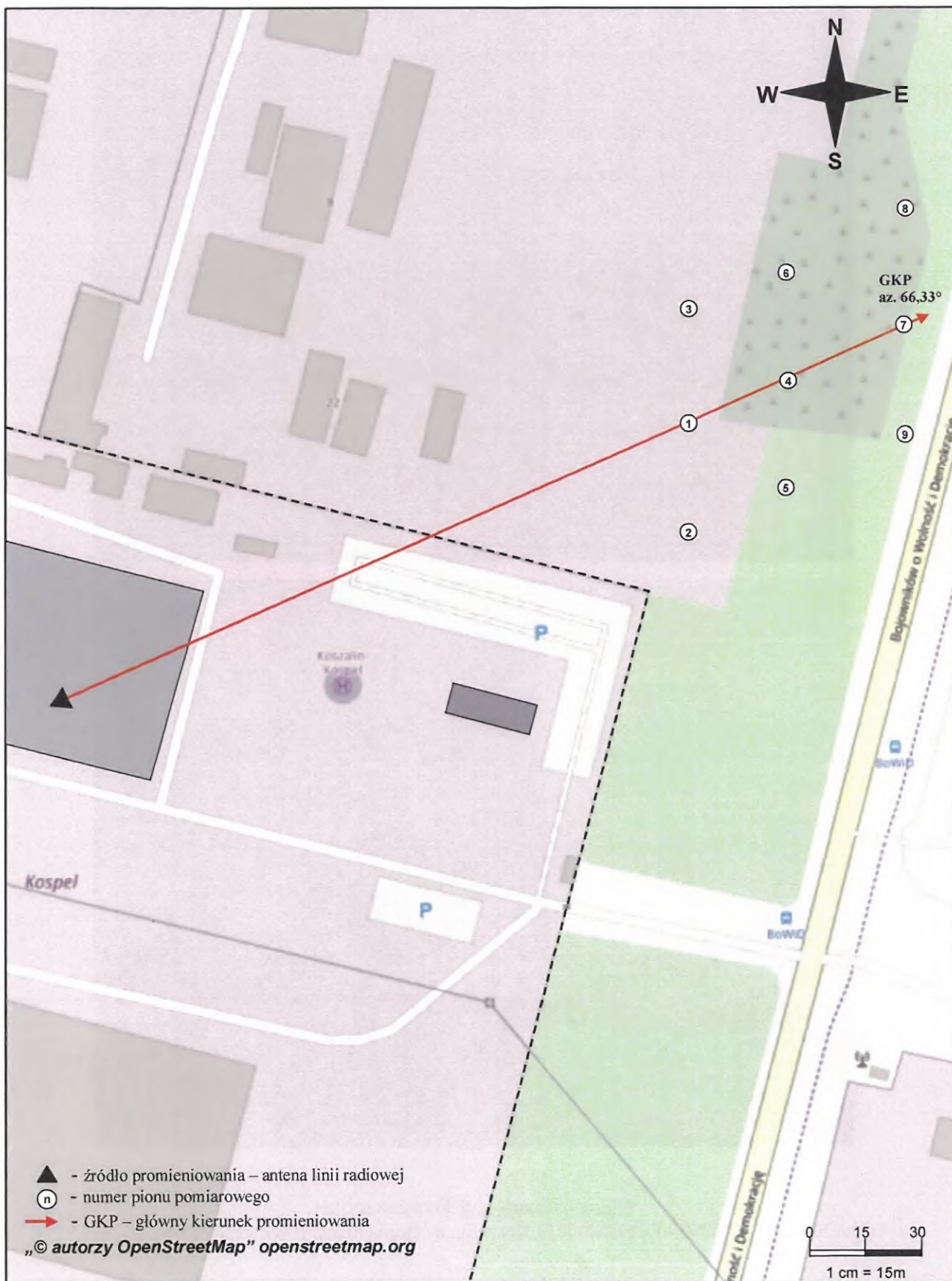
Rys. 1. Usytuowanie punktów i pionów pomiarowych w otoczeniu instalacji radiokomunikacyjnej Stacja Netia KOSZB090-KOSZM00033 Koszalin, ul. Bojowników o Wolność i Demokrację 24
