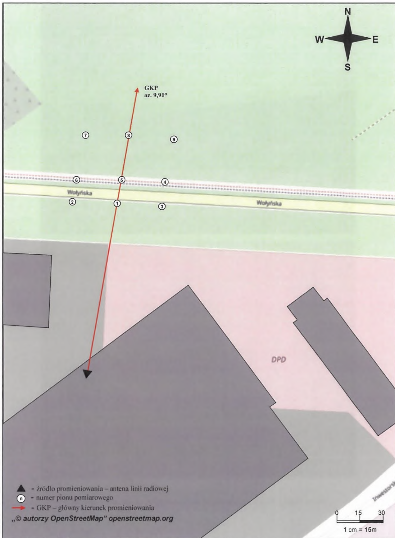
Rys. 1. Usytuowanie punktów i pionów pomiarowych w otoczeniu instalacji radiokomunikacyjnej Stacja Netia KOSZB196-KOSZM00032 Koszalin, ul. Ekonomiczna 20
