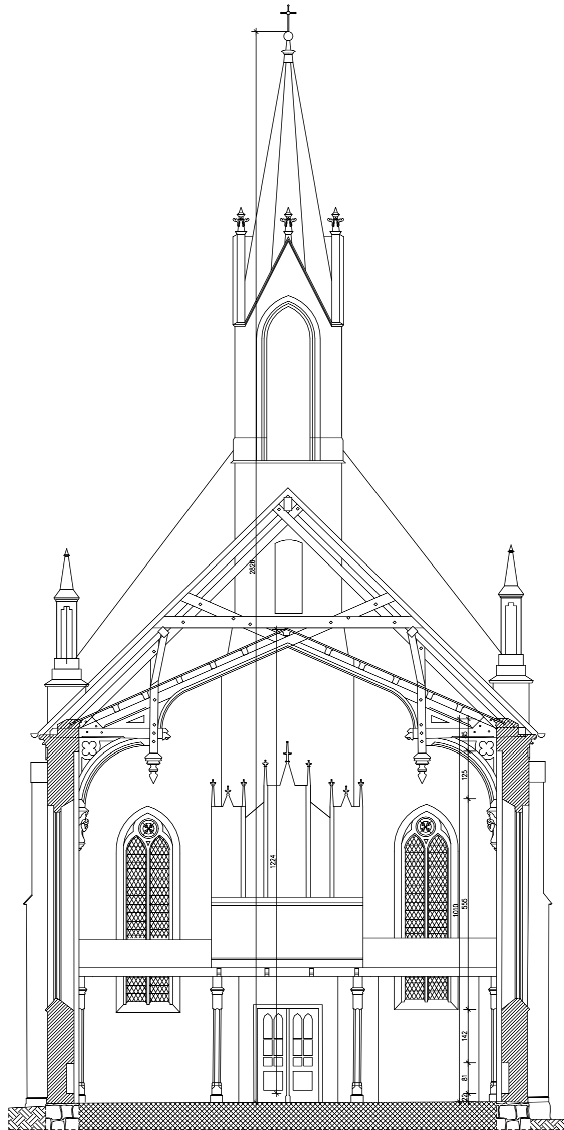
Przekrój B-B
